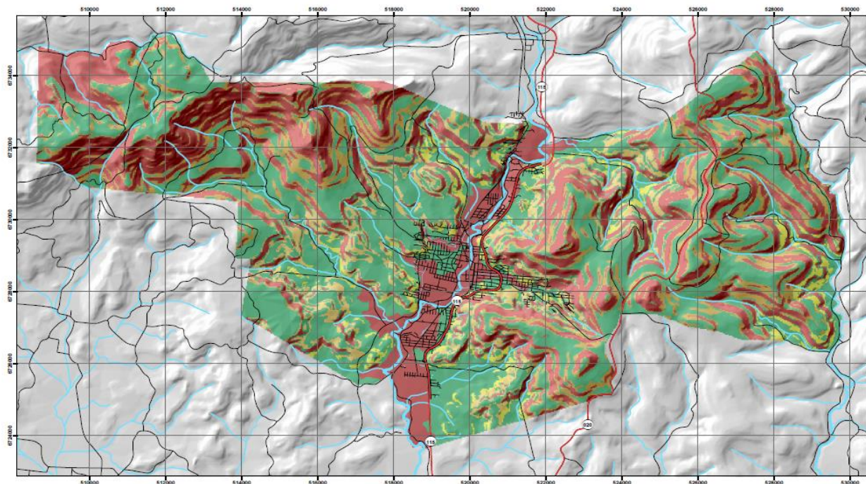
CARTA GEOTÉCNICA DE SUSCETIBILIDADE A ESCORREGAMENTOS E INUNDAÇÕES DO MUNICÍPIO DE IGREJINHA incorporando sombreamento de terreno
